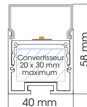
Diffuseur en U 18 mm
