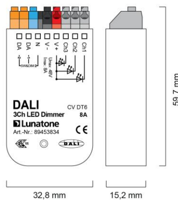
dimensions back box Version 8A Art.Nr.: 89453834 Version 4A Art. Nr.: 89453828
